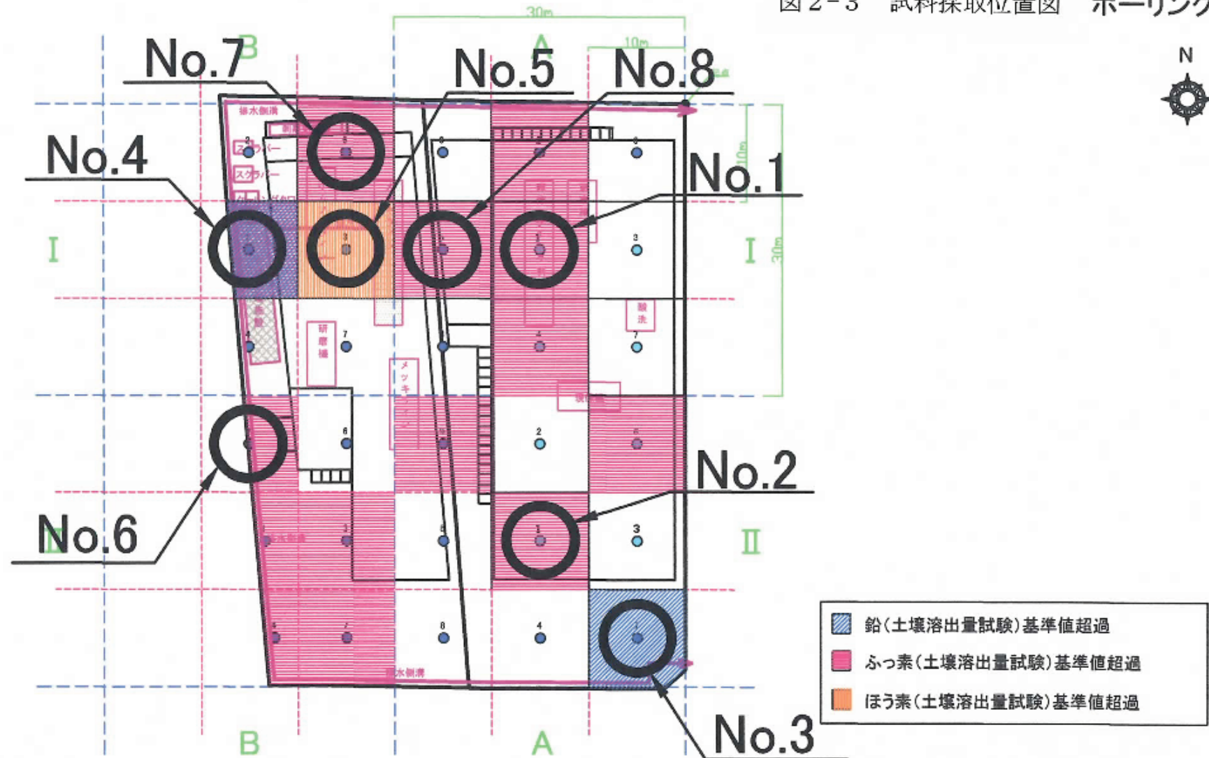
図2-3 試料採取位置図 ボーリングエ
