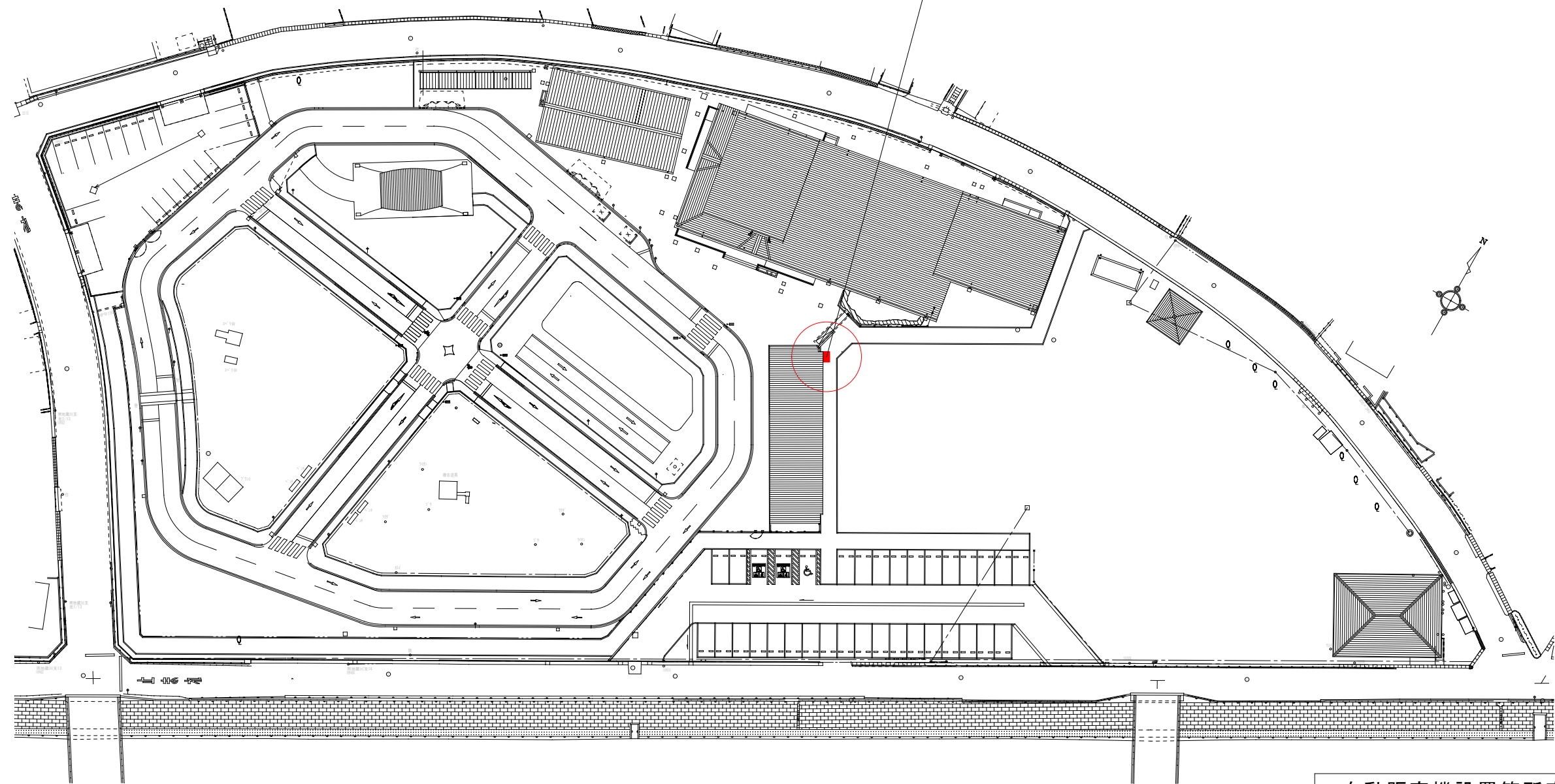
配置図
