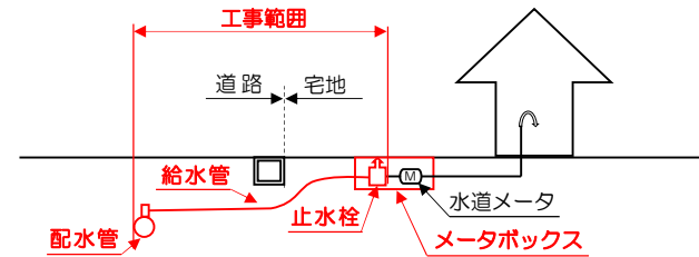
工事範囲イメージ図
