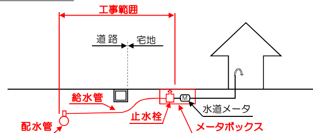
工事範囲イメージ図
