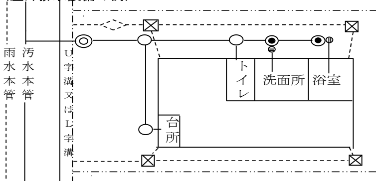
(屋外排水設備の例)
