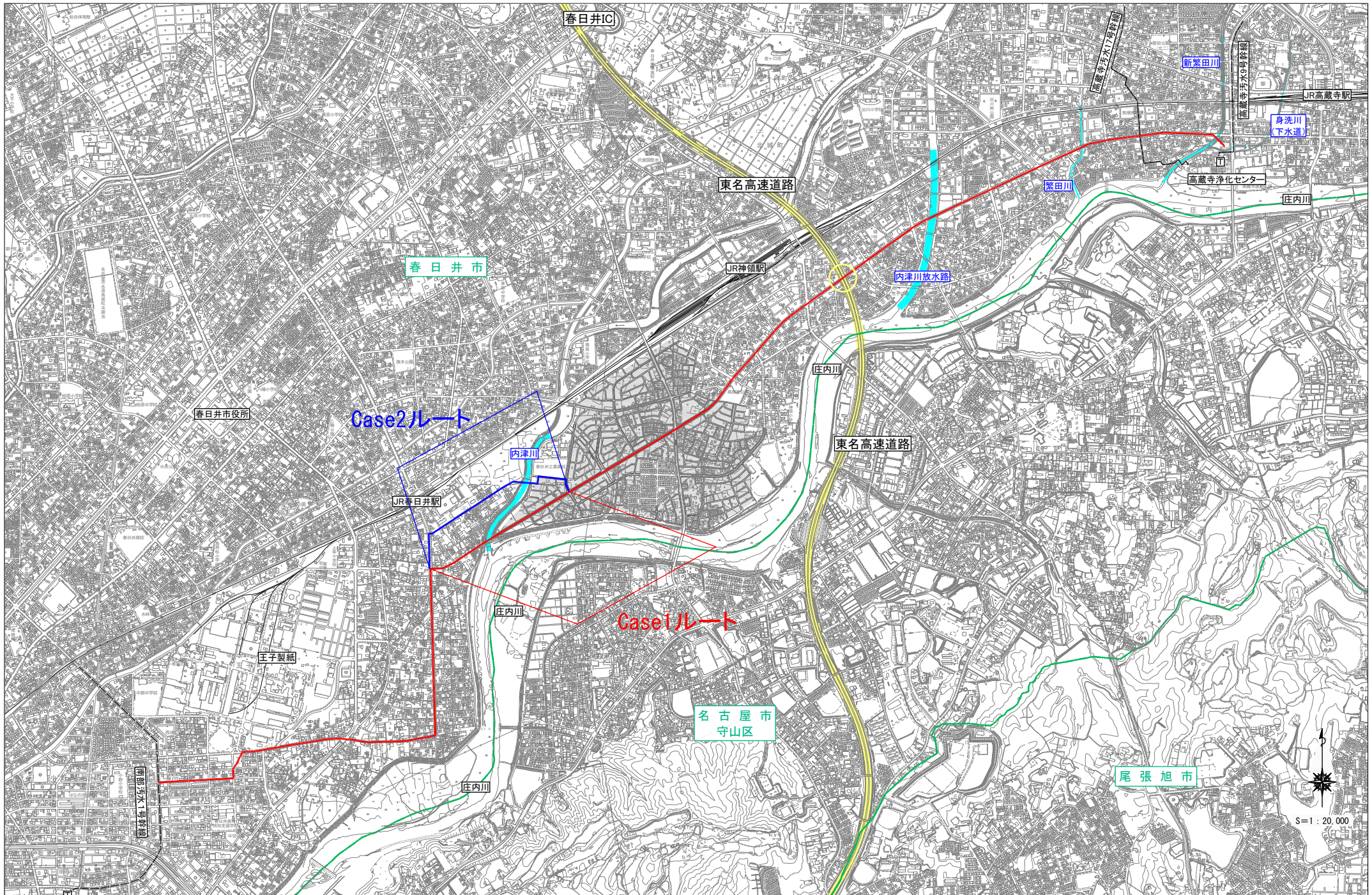
接続管平面図
