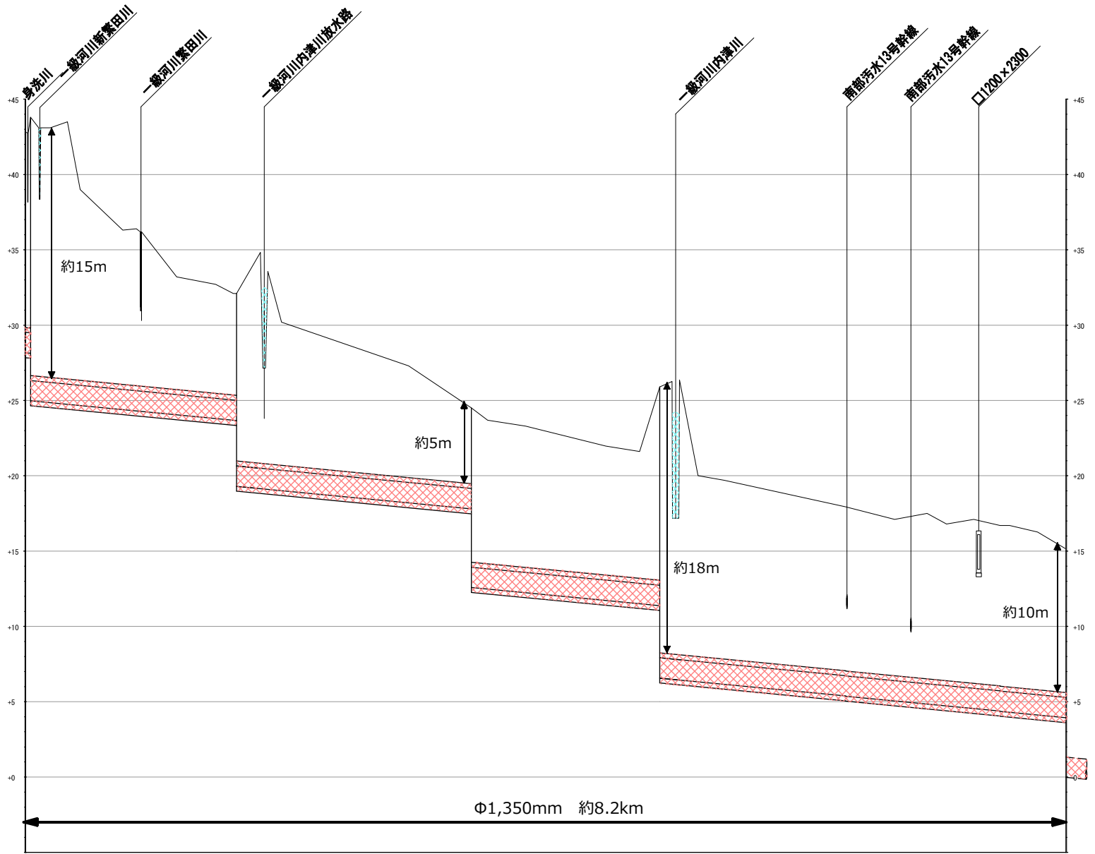
接続管縦断図 (Case 1 ルート)
