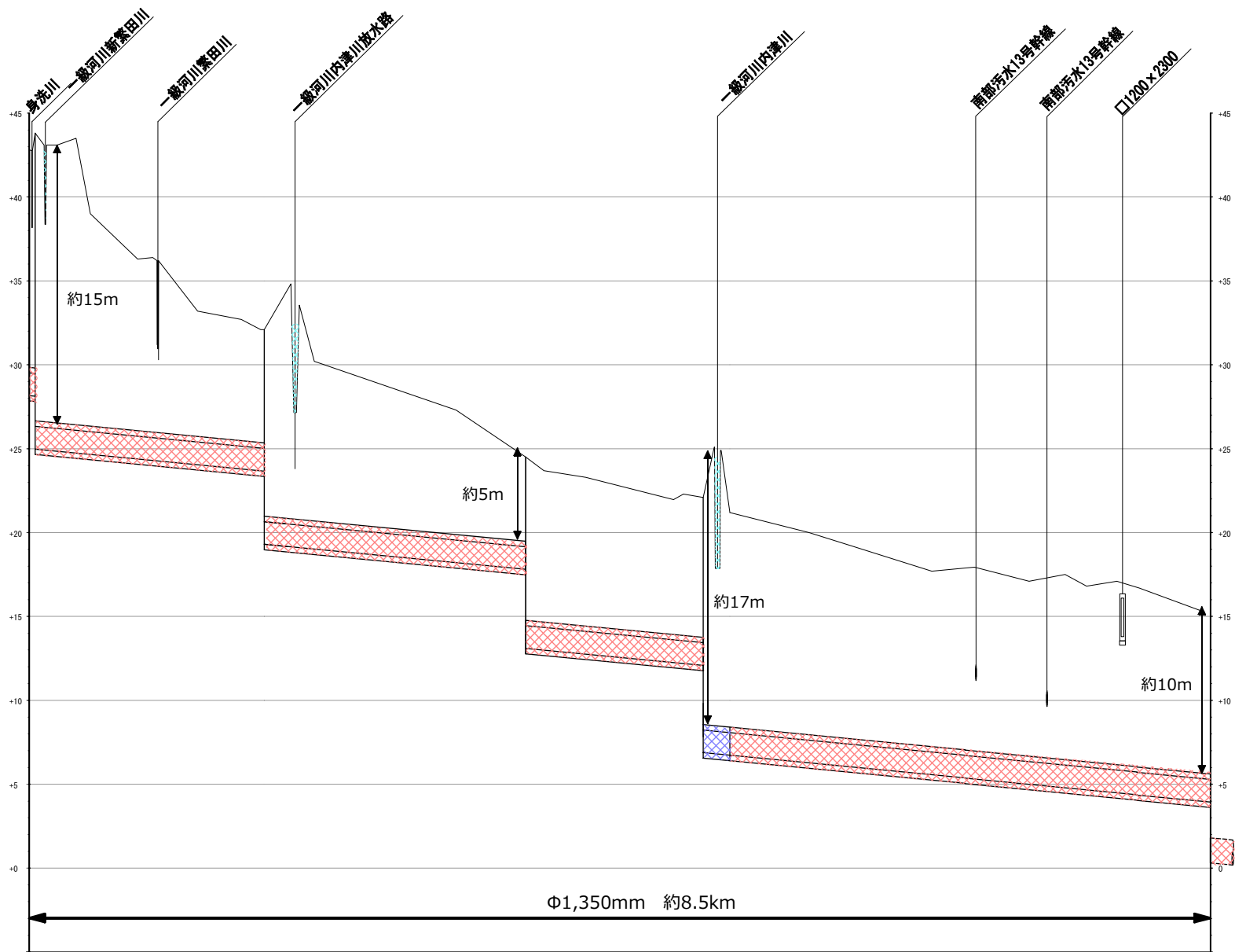
接続管縦断図 (Case 2 ルート)
