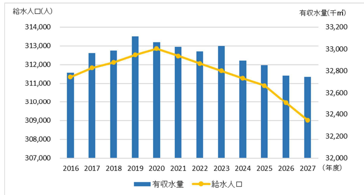
【給水人口と有収水量の推計】
