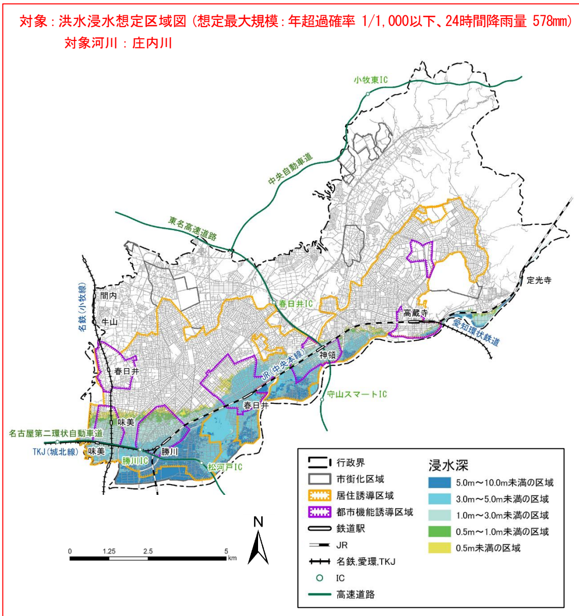
【図 8-5 庄内川の想定最大規模降雨による洪水の浸水深（洪水浸水想定区域図）】
