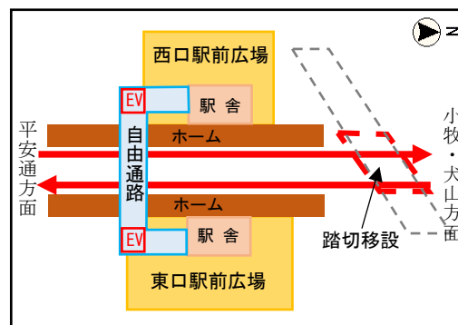
計画図
