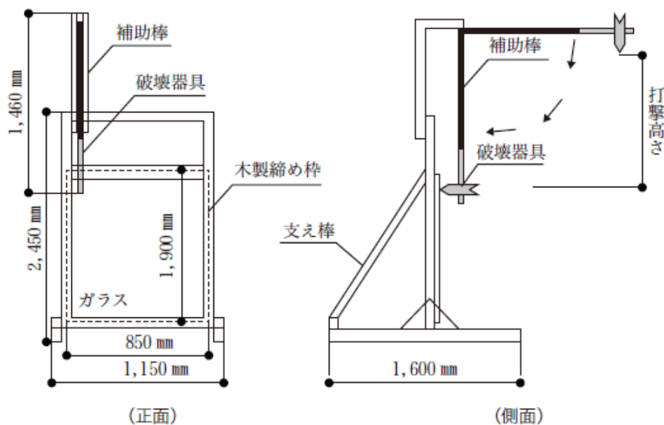
図1 本体
