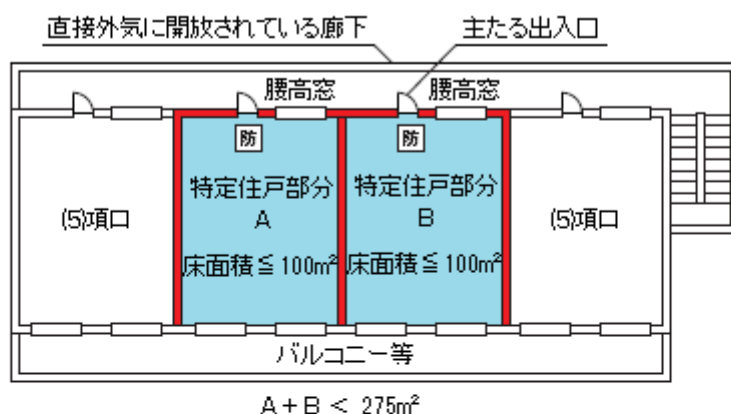
(特定住戸部分拡大図)
