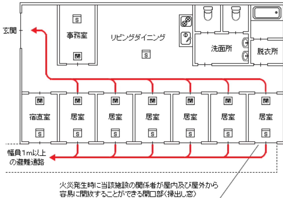
別図5 省令第12条の2第2項第2号
