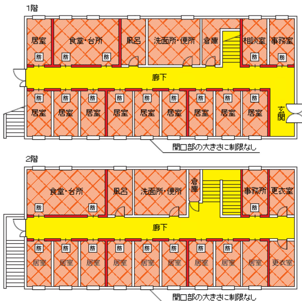
別図2 省令第12条の2第1項第1号
