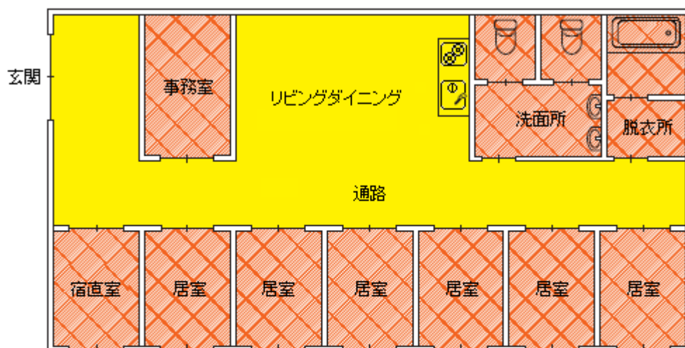
別図4 省令第12条の2第2項第1号
