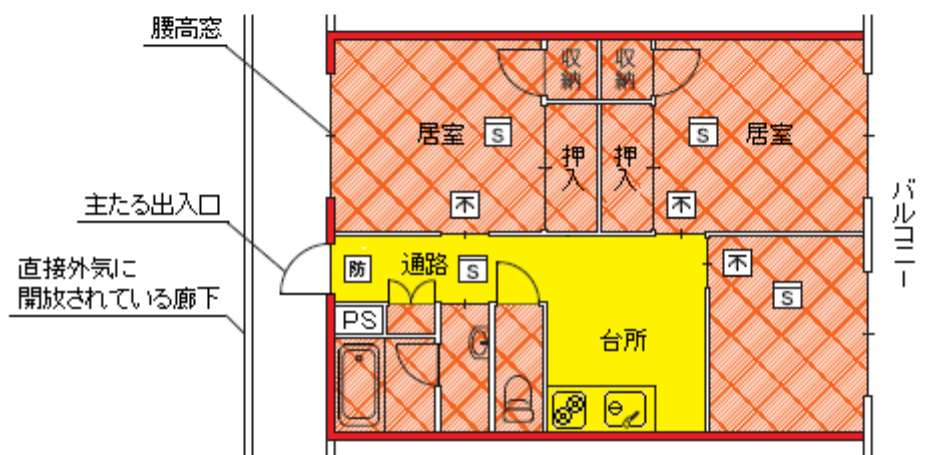
(特定住戸部分拡大図)
