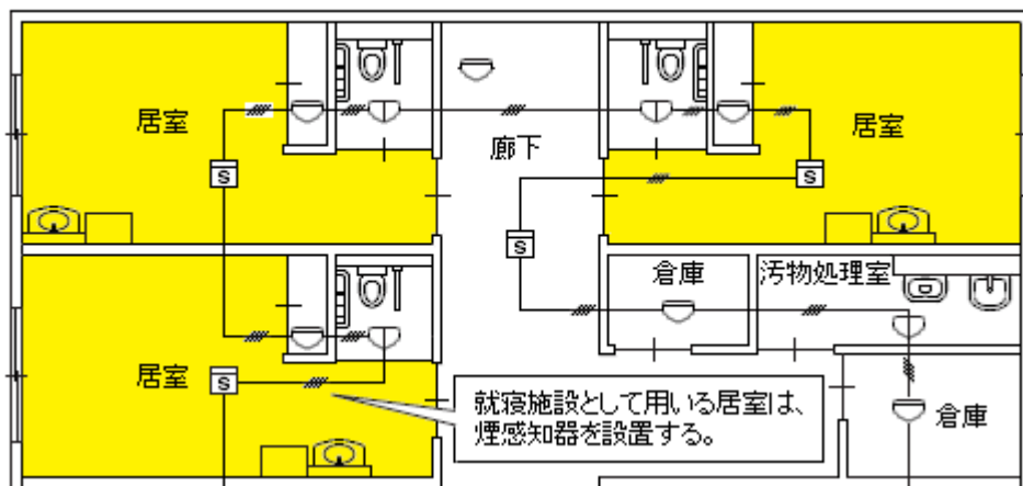
（政令別表第1(6)項口に掲げる防火対象物（無窓階以外の階）の例）
