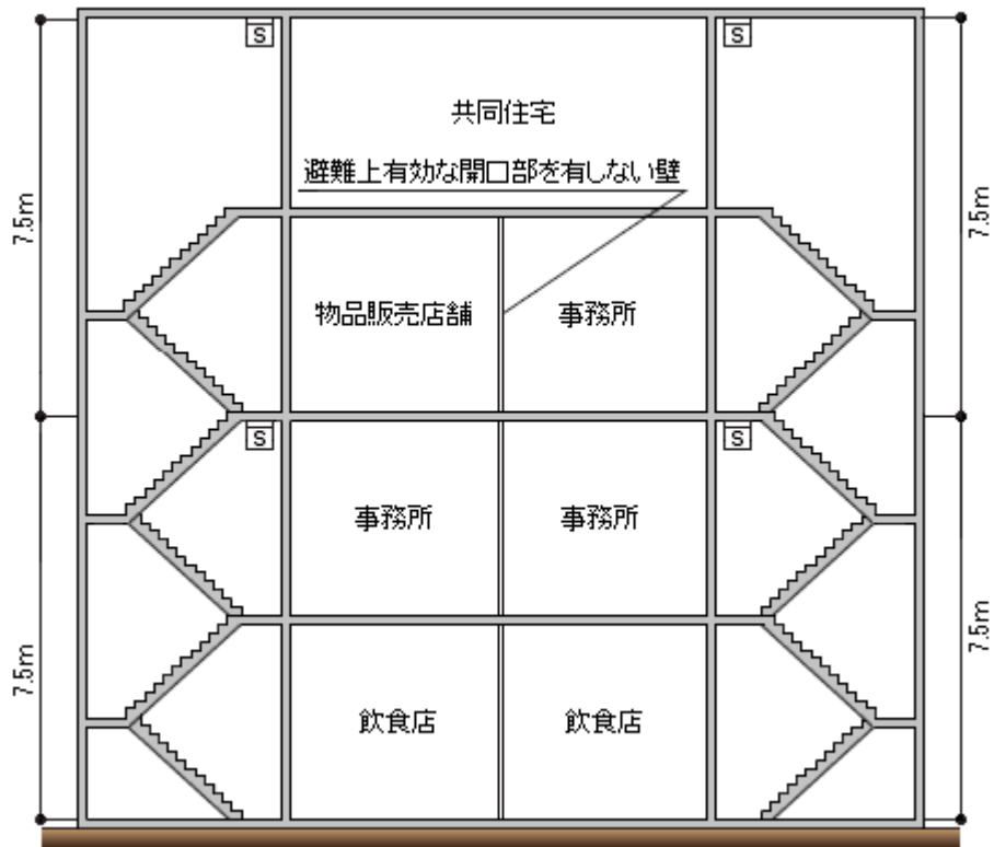
(特定一階段等防火対象物の例 その3)
