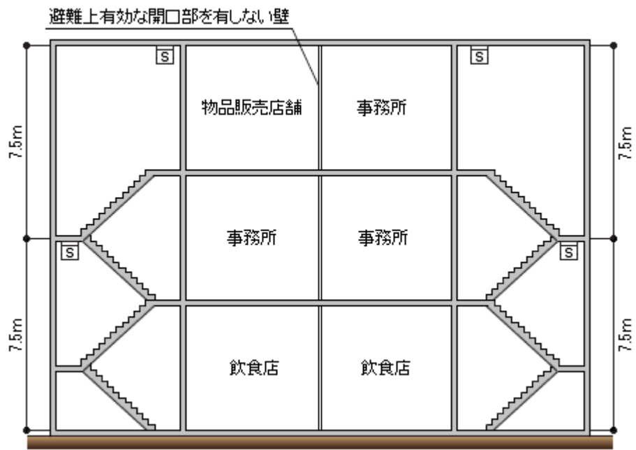
(特定一階段等防火対象物の例 その1)
