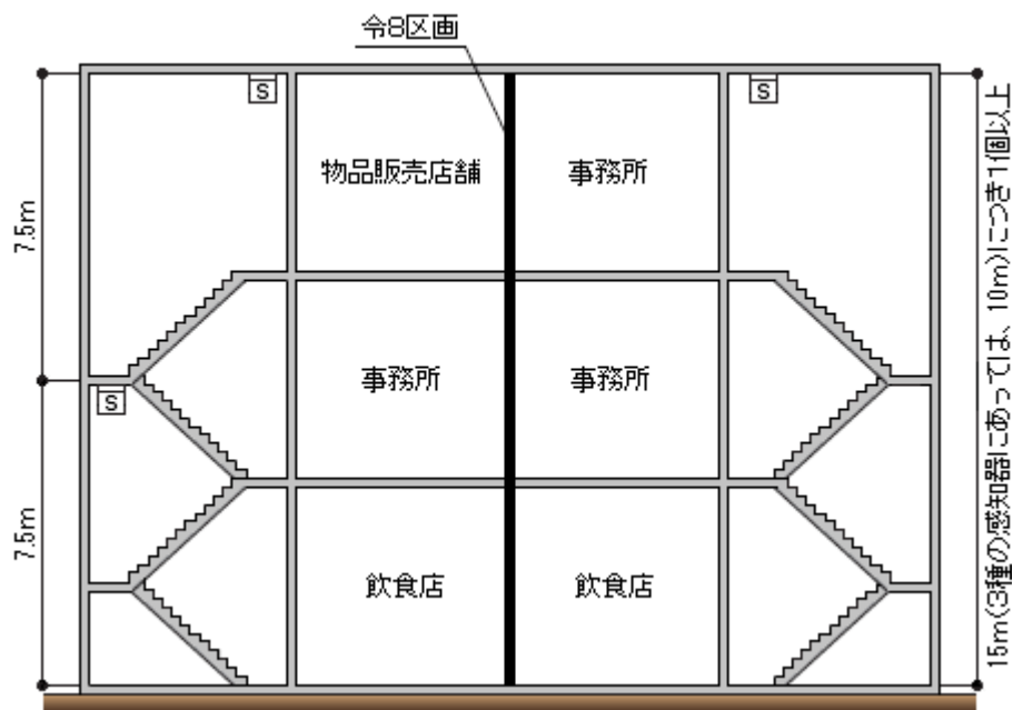
(特定一階段等防火対象物の例 その2)
