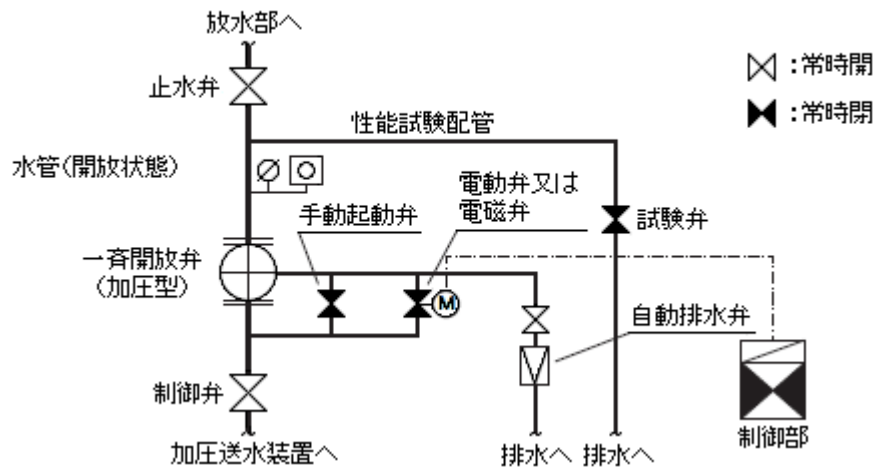
(減圧方式の一斉開放弁等周りの配管の例)
