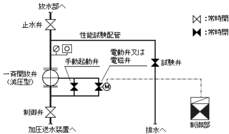
(加圧方式の一斉開放弁等周りの配管の例)
