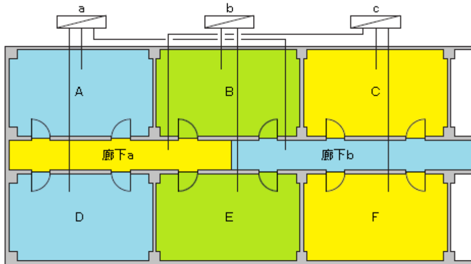
(隣接する同時放射区域の考え方及び防護区画の組み合わせの例)
