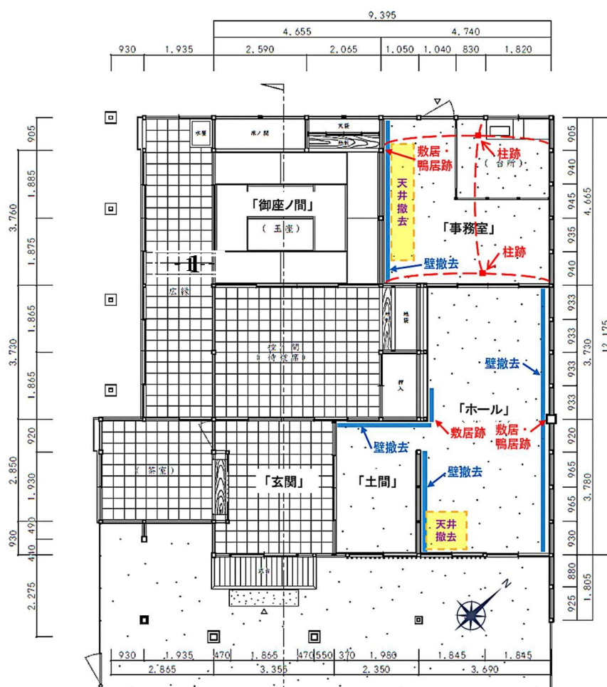
図 - 1 解体前 取り解き調査図
